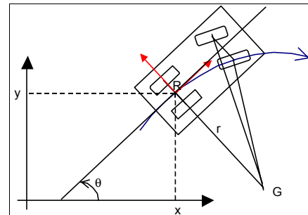
Fig. 1 – Modelo do veículo.
