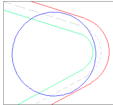
Fig. 7 – Exemplo de troço de curva simples.
