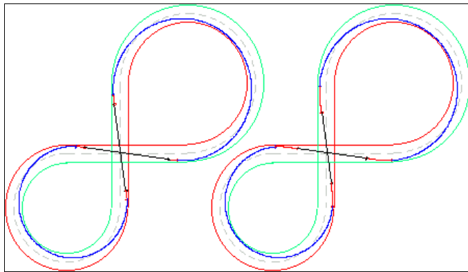
Fig. 11 – Exemplos de variação da margem m .
