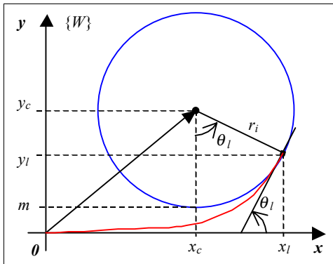
Fig. 3 – Modelo para cálculo de uma clotóide.
