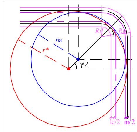
Fig. 5 – Circunferências de maior raio e de apoio média.
