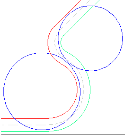
Fig. 8 – Exemplo de troço de curva contra-curva.
