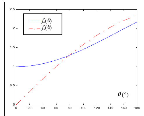
Fig. 4 – Gráficos de funções invariantes do algoritmo.
