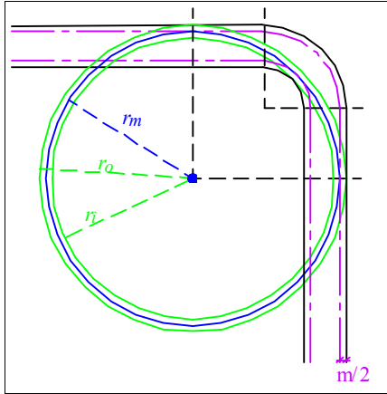
Fig. 6 – Circunferências de apoio interior, exterior e média.
